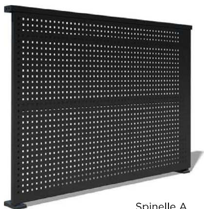
Spinelle A
